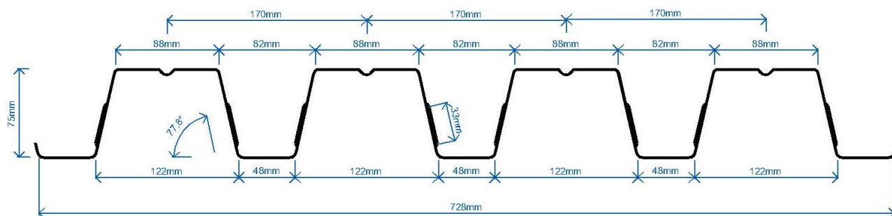
Εικόνα 1: Ονομαστικές διαστάσεις του τραπεζοειδούς χαλυβδόφυλλου CYDECK 75.
