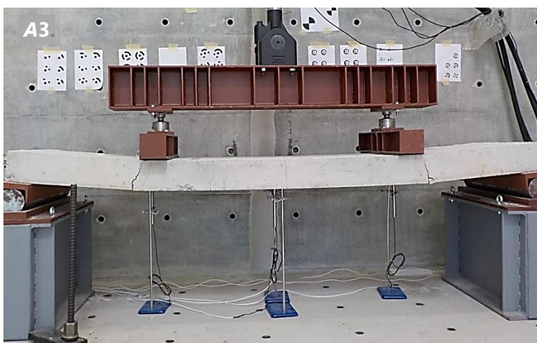
Εικόνα 5: Ρηγμάτωση και ακραία ολίσθηση στην αστοχία που καταγράφηκαν κατά τον πειραματικό έλεγχο των δοκιμών σειράς Α. Σύμμικτες πλάκες Α1 (α), Α2 (β) και Α3 (γ).
