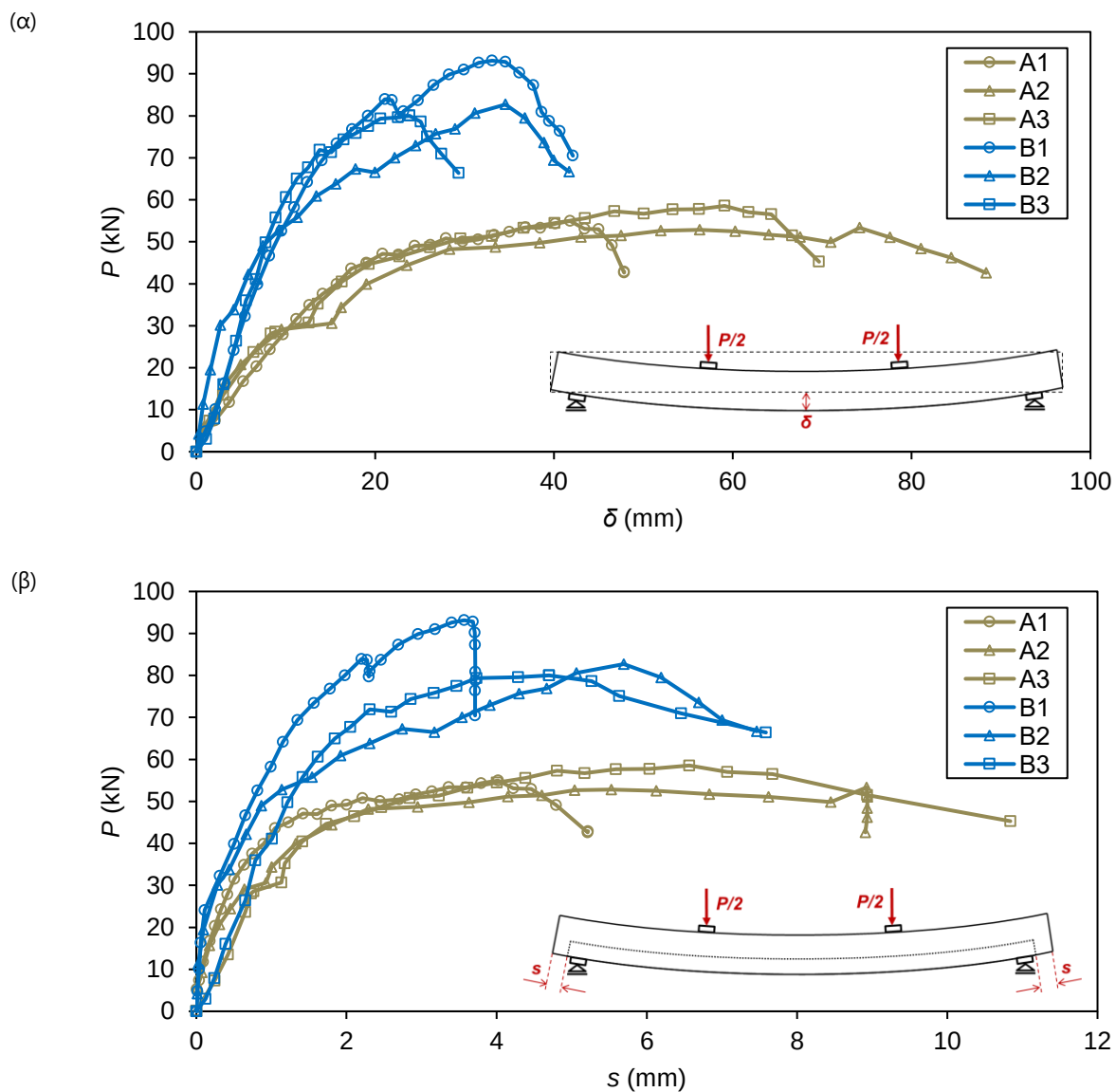
Εικόνα 4: Διαγράμματα (α) επιβαλλόμενης δύναμης P - βύθισης στο κέντρο της κάτω ίνας \delta της κάθε πλάκας και (β) επιβαλλόμενης δύναμης P - μέσης ολίσθησης στα δυο άκρα s της κάθε πλάκας που πρόεκυψαν από τον πειραματικό έλεγχο έξι πλακών με δύο διαφορετικά διατμητικά ανοίγματα.
