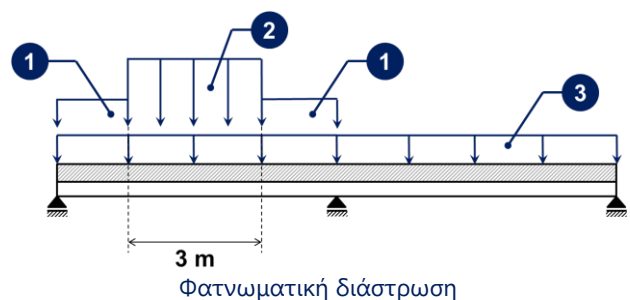
Συνεχής πλάκα δυο ανοιγμάτων
