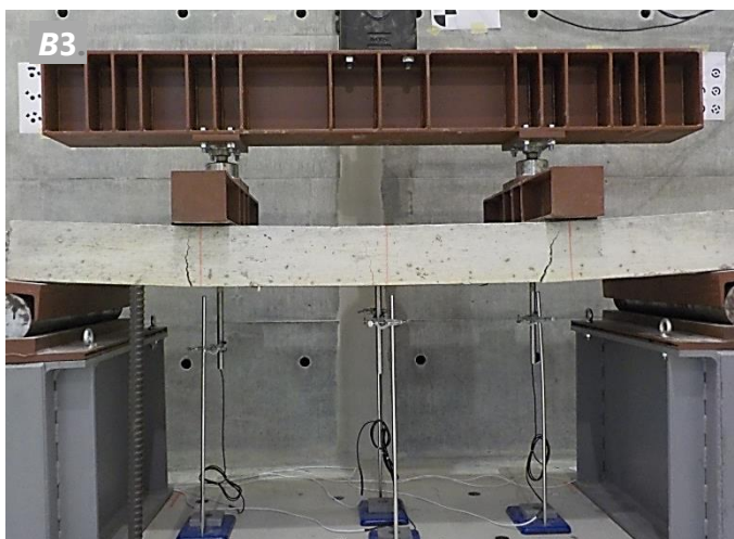
Εικόνα 6: Ρηγμάτωση και ακραία ολίσθηση στην αστοχία που καταγράφηκαν κατά τον πειραματικό έλεγχο των δοκιμών σειράς Β. Σύμμικτες πλάκες B1 (α), B2 (β) και B3 (γ).
